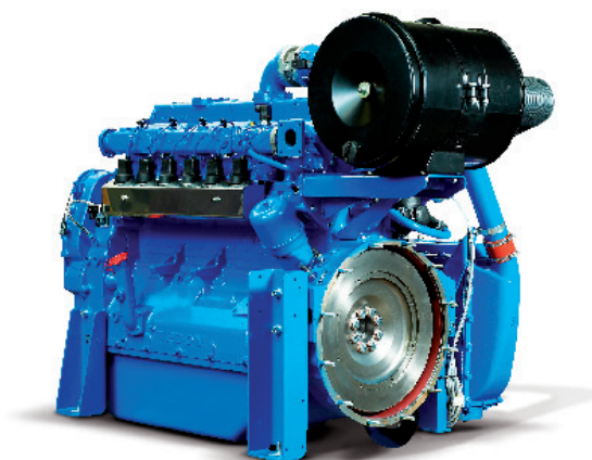
Motor TEDOM s výkonovým rozsahem 80–200 kW
